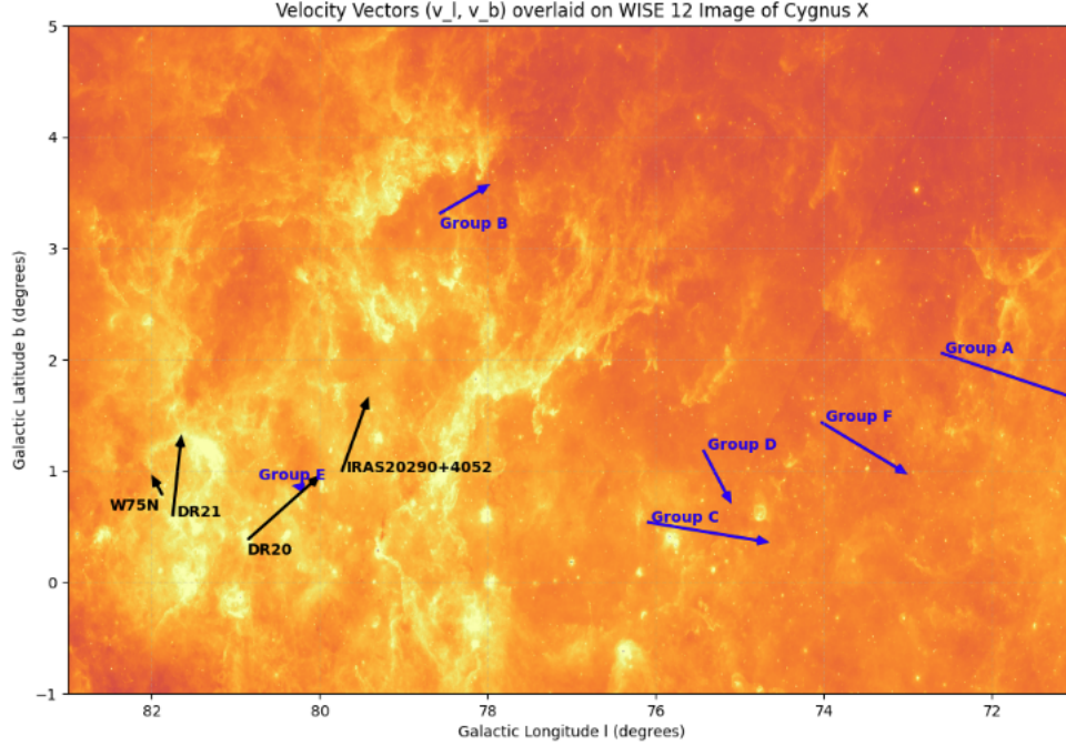
FIGURE 6 – Projection des vitesses v_l et v_b des nuages moléculaires et des groupes d'étoiles massives sur une image WISE à 12 \mu m. L'abscisse est la longitude galactique et l'ordonnée est la latitude galactique. Les nuages moléculaires sont en noir et les groupes d'étoiles en bleu
